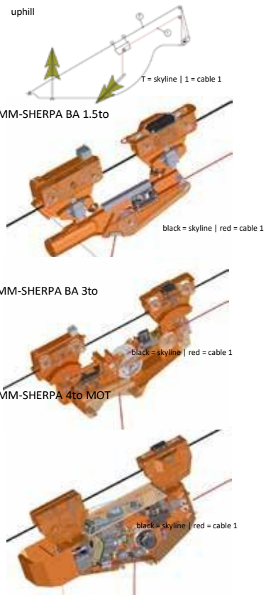
MM-SHERPA BA® 2-Vaersystem (Vinsjing Oppover) 1.5to / 3to / 4to
